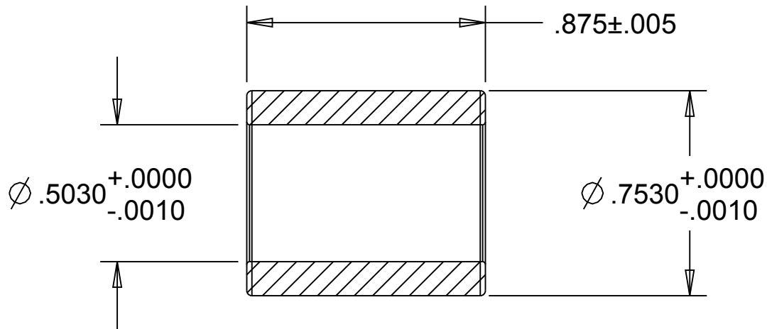
SECTION A-A
