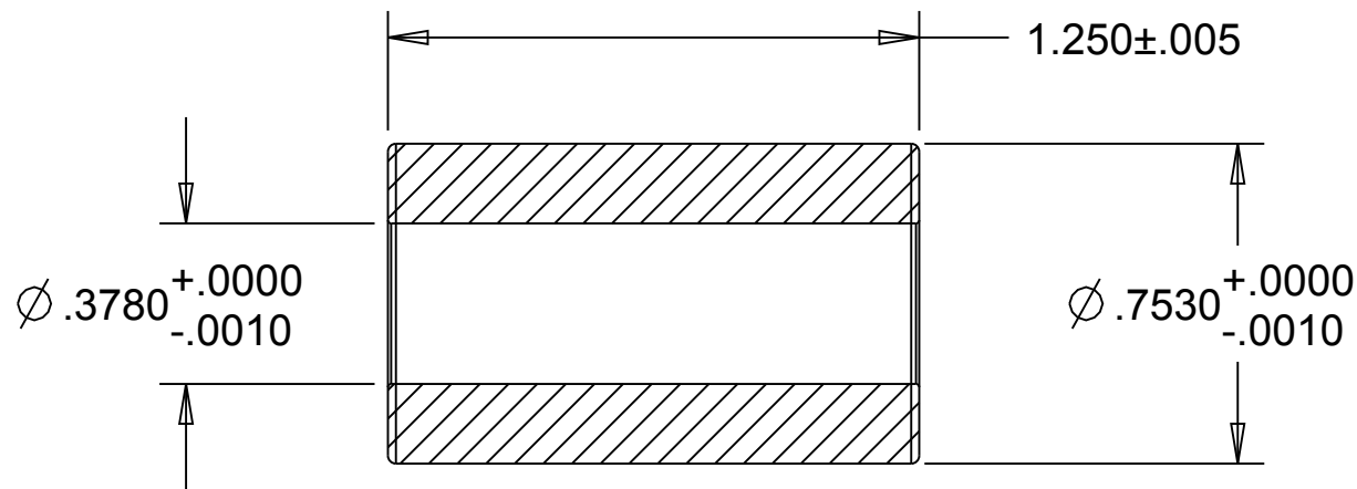
SECTION A-A
