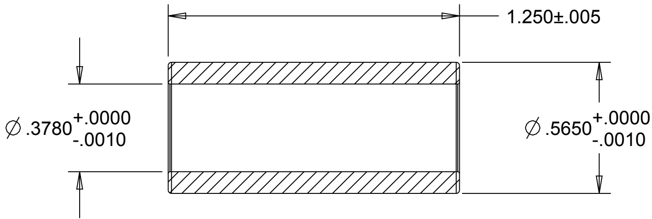
SECTION A-A
