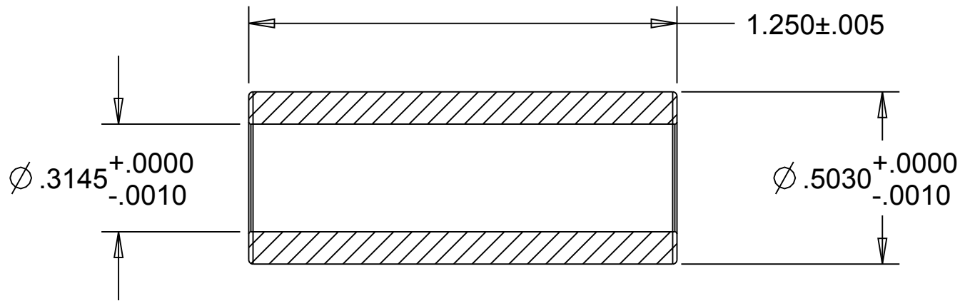
SECTION A-A
