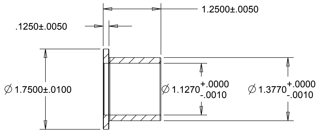
SECTION A-A
