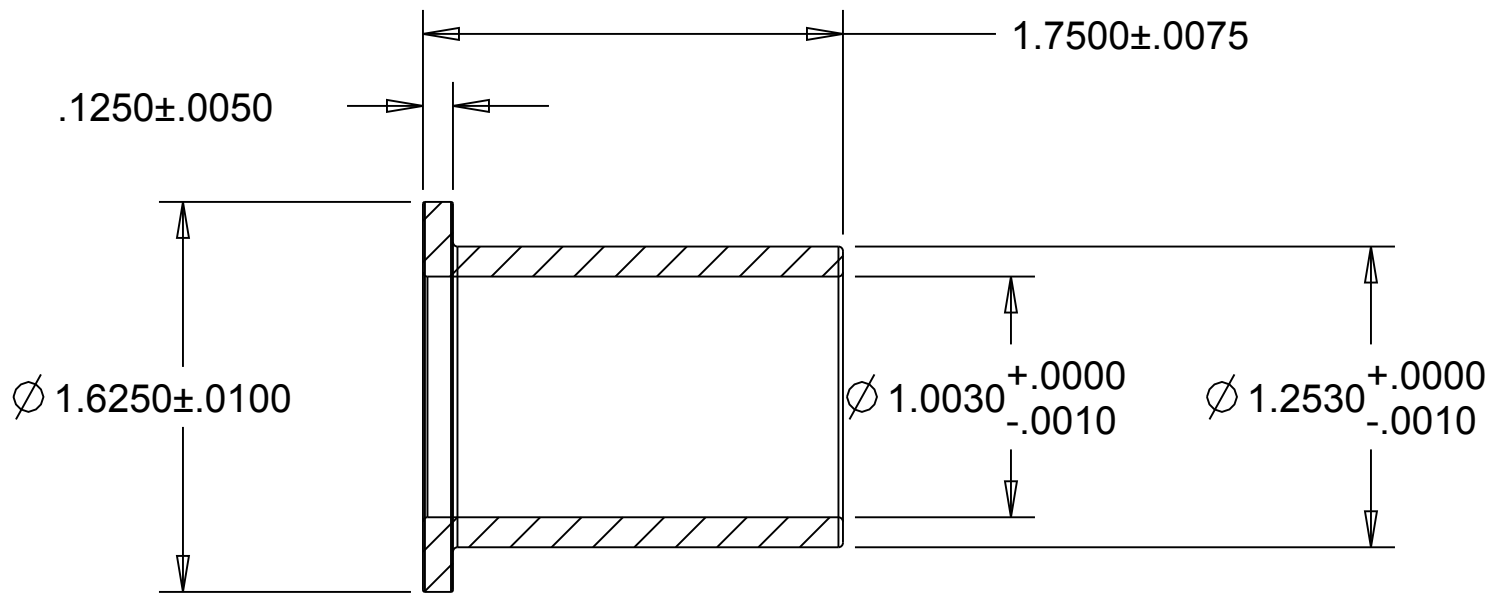
SECTION A-A
