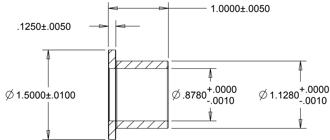
SECTION A-A
