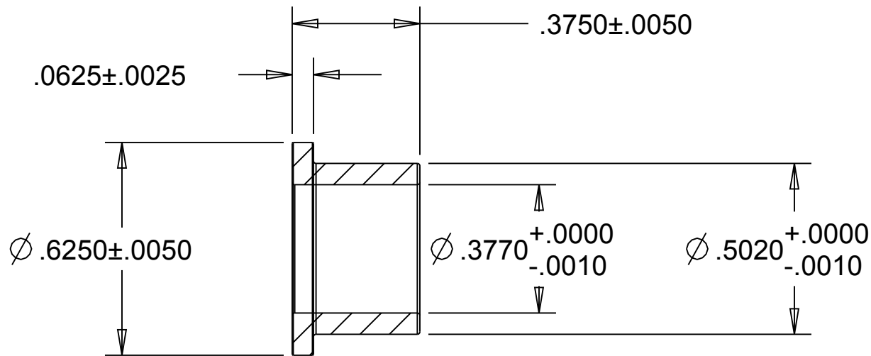
SECTION A-A
