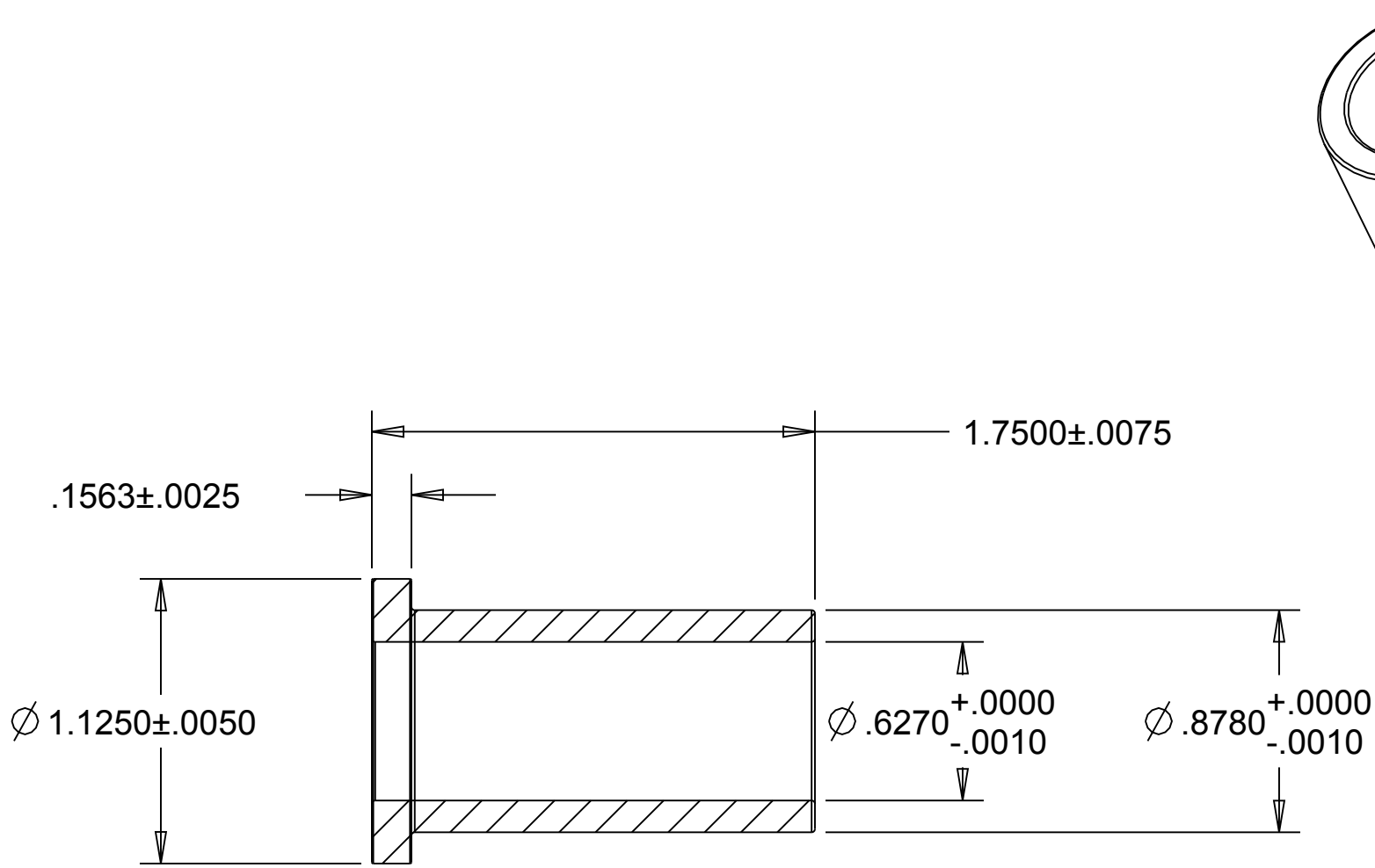
SECTION A-A
