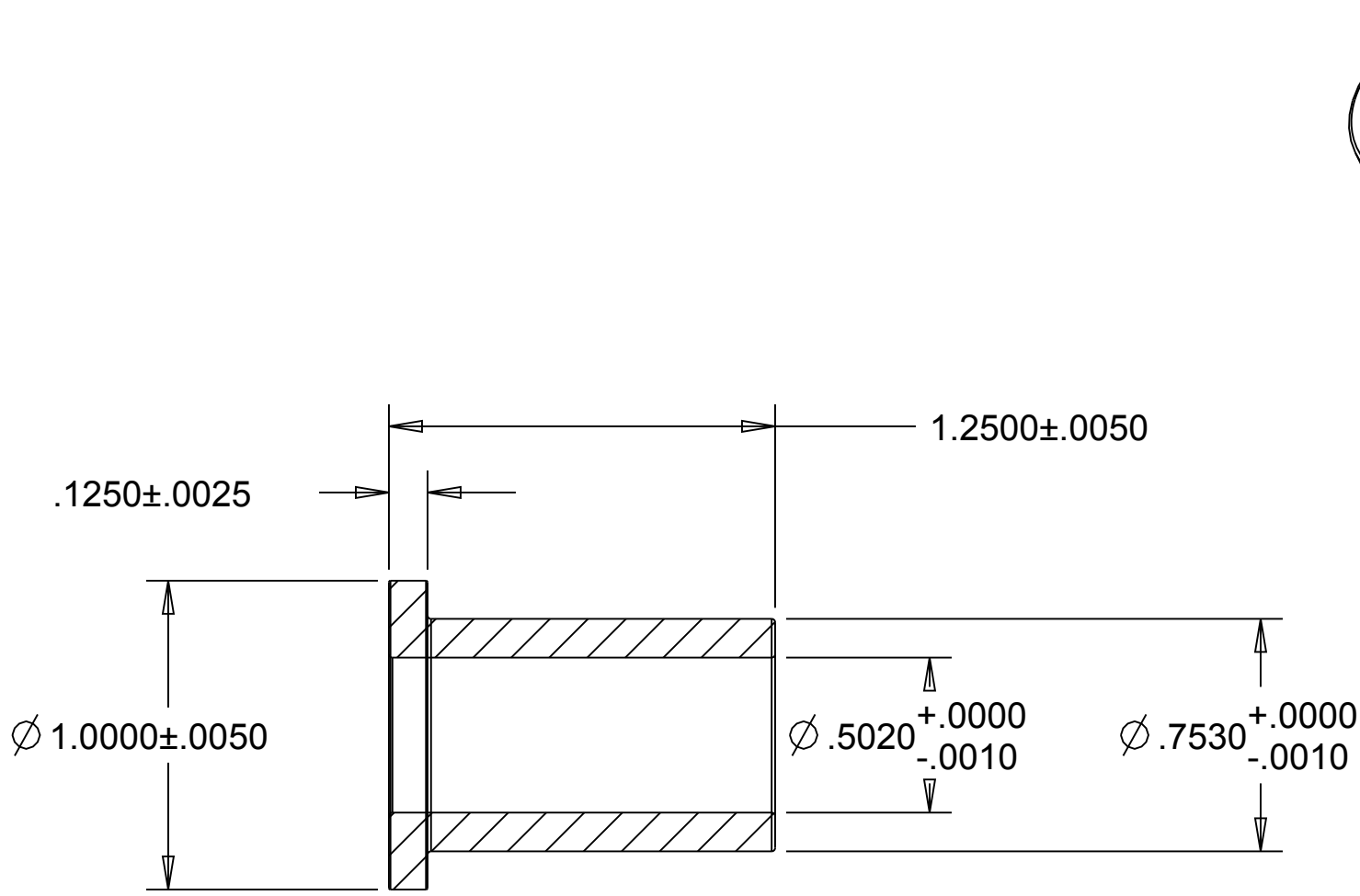
SECTION A-A
