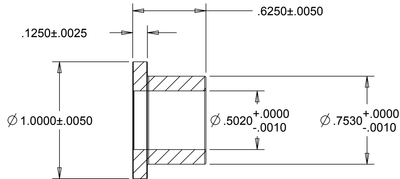
SECTION A-A
